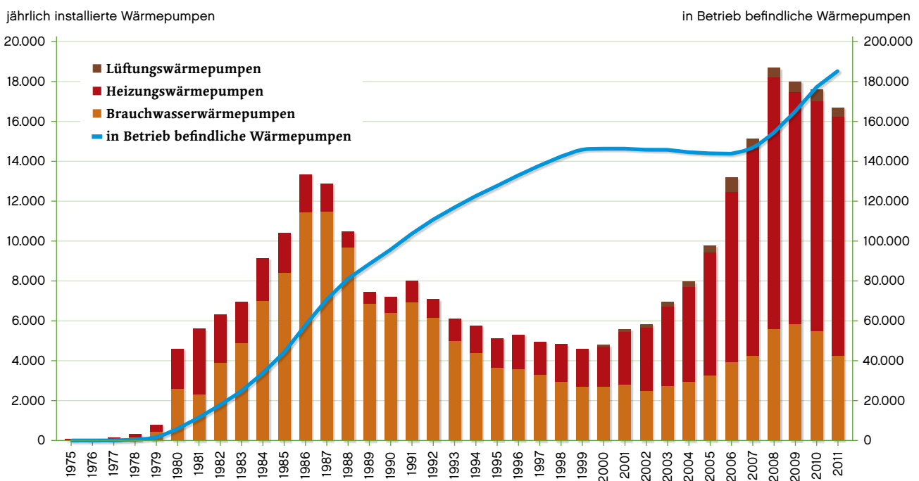
Abb. 7.6 | Wärmepumpen in Österreich 1975-2011
