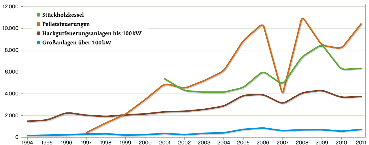
Abb. 7.1 | Jährlich installierte Biomasse-Heizungen 1994-2011
