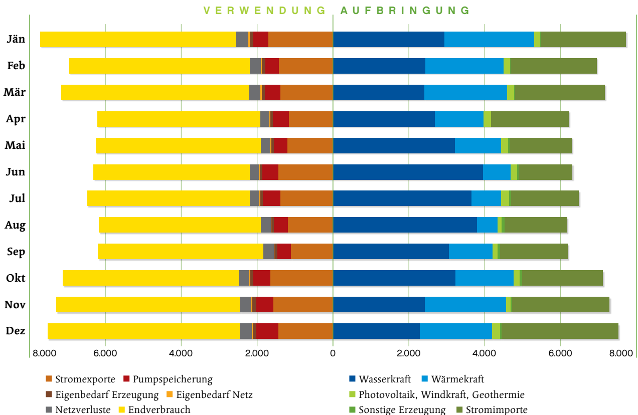
Abb. 4.3 | Jahresbilanz elektrischer Strom nach Monaten
