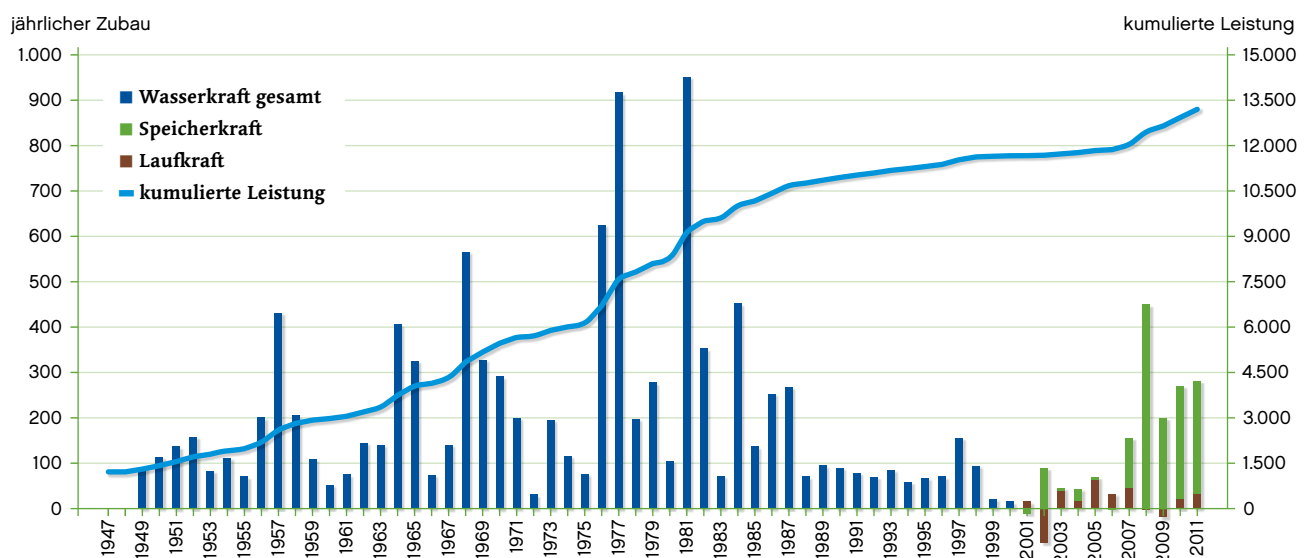
Abb. 7.7 | Wasserkraftwerke in Österreich 1948-2011
