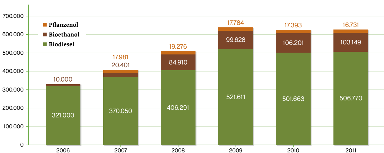
Abb. 7.2 | Jährlich abgesetzte Biotreibstoffe 2006-2011
